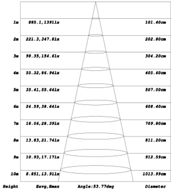
Beam angle: 55°
